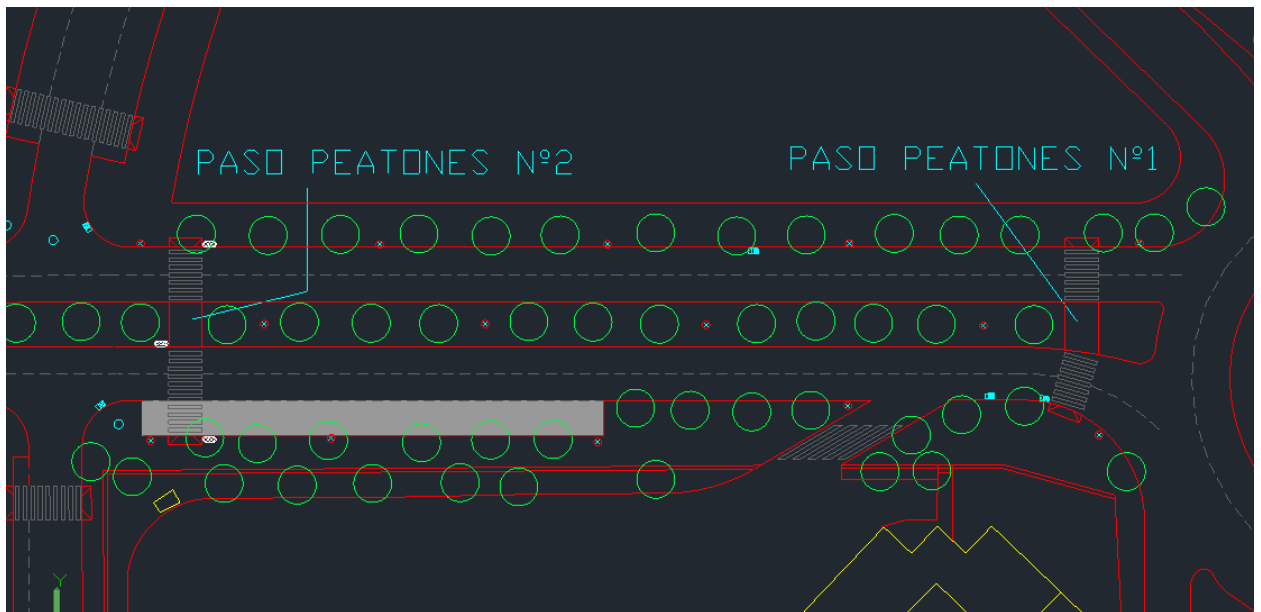
Diseño actual Pasos de Peatones nº 1 y nº 2
